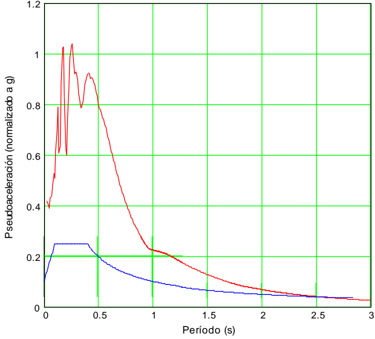
ESPECTRO TERREMOTO DE LORCA
