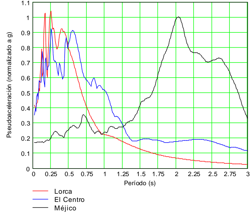
ESPECTROS DE RESPUESTA
